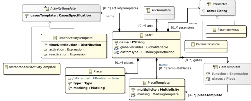
Fig. 3. SAN-T metamodel — Core .
