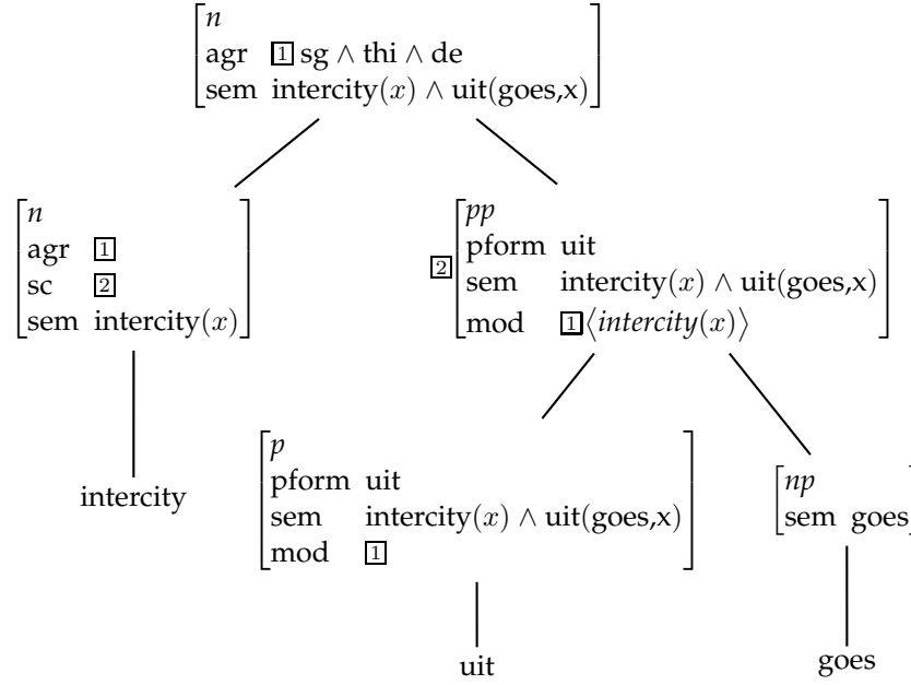
Figure 5: intercity uit Goes (intercity from Goes)
