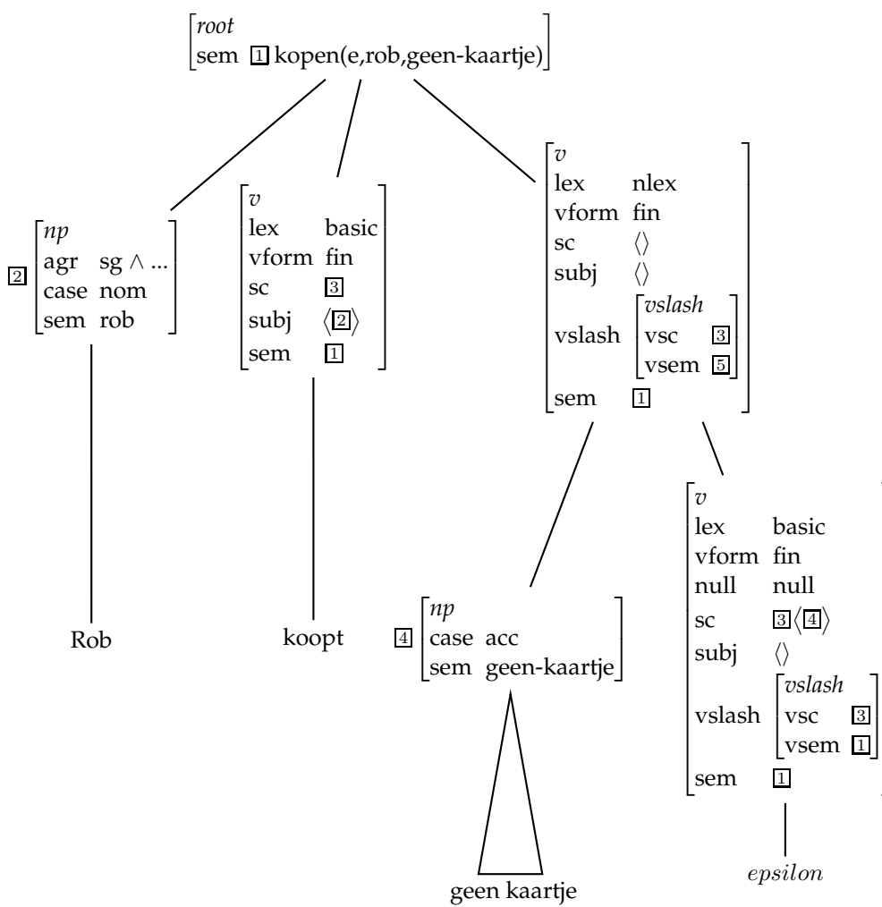
Figure 11: Rob koopt geen kaartje (Rob does not buy a ticket)
