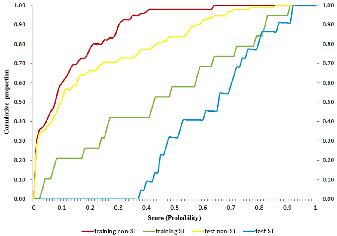
Figure 2 Kolmogorov-Smirnov Plots
