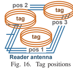
Fig. 16. Tag positions
