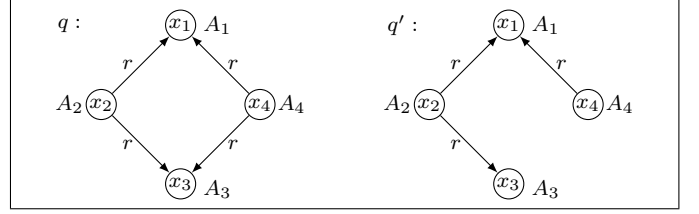
Fig. 2. CQs for Example 1
