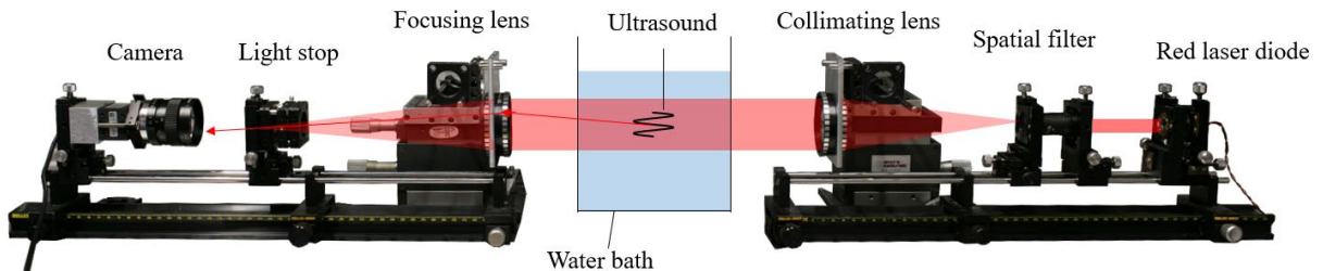
Fig. 2. Pulsed laser schlieren setup
