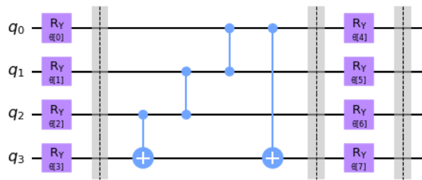
Fig. 9. Circuit 4
