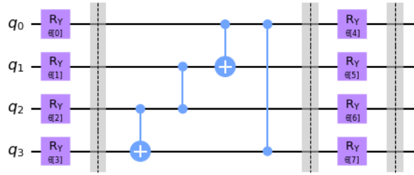
Fig. 8. Circuit 3
