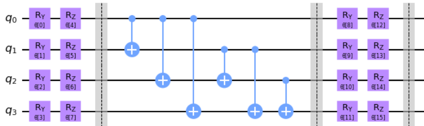
Fig. 17. Circuit 12
