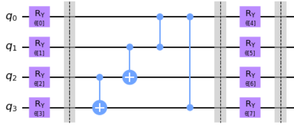
Fig. 10. Circuit 5
