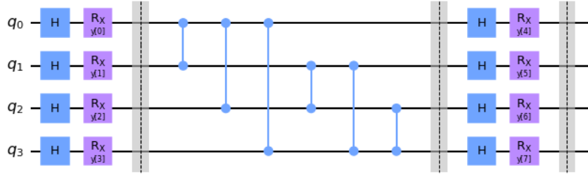
Fig. 15. Circuit 10
