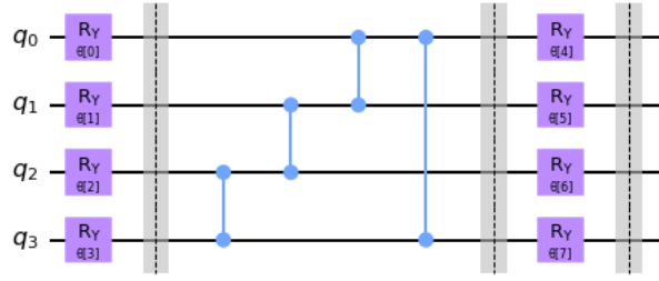
Fig. 7. Circuit 2
