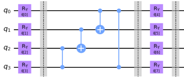
Fig. 12. Circuit 7
