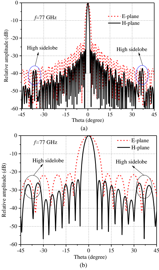
Fig. 6. Synthesized radiation patterns. (a) 16x32 subarray antenna; (b) 4x8 subarray antenna.
