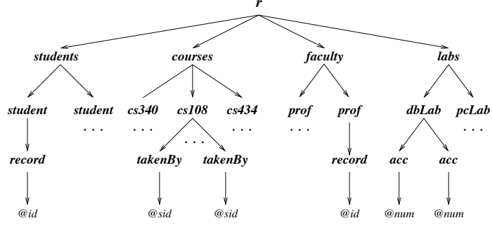
FIG. 1.1. An XML document.
