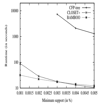
Fig. 21. Runtime comparison( T10I4D100K ).
