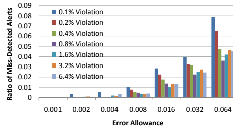
Figure 45: Actual Mis-Detection Rates
